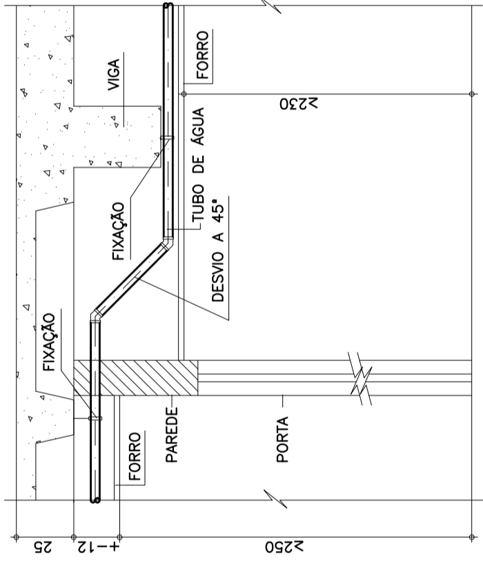
CORTE AA - DESVIO SOB A VIGA NO HALL DOS ELEVADORES SEM ESCALA
